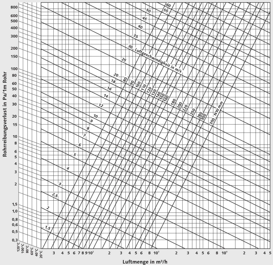
Diagramm Rohrreibungsverlust
