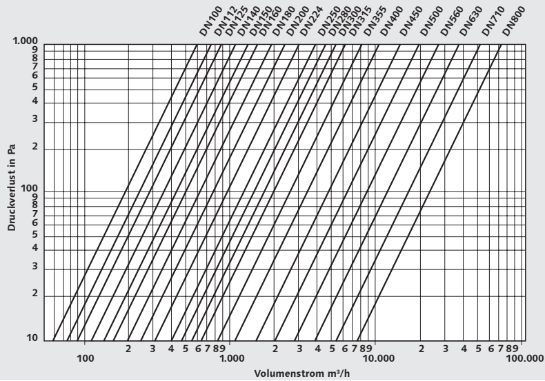
Diagramm Druckverlust
